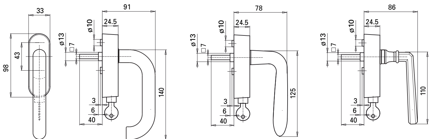
Maße Sperrteil, gilt für alle Modelle
